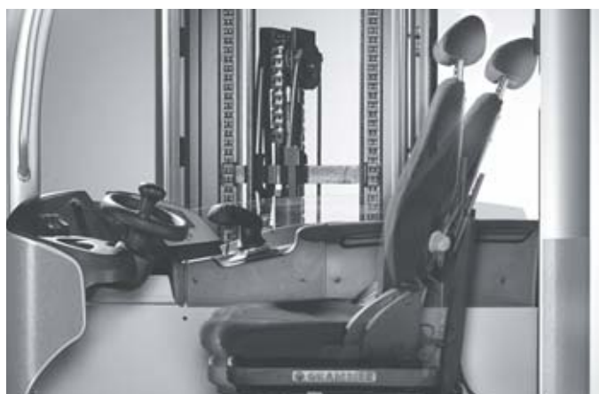
Ampia visibilità anche con carichi sulle forche, grazie all'esclusivo e confortevole sedile reclinabile
